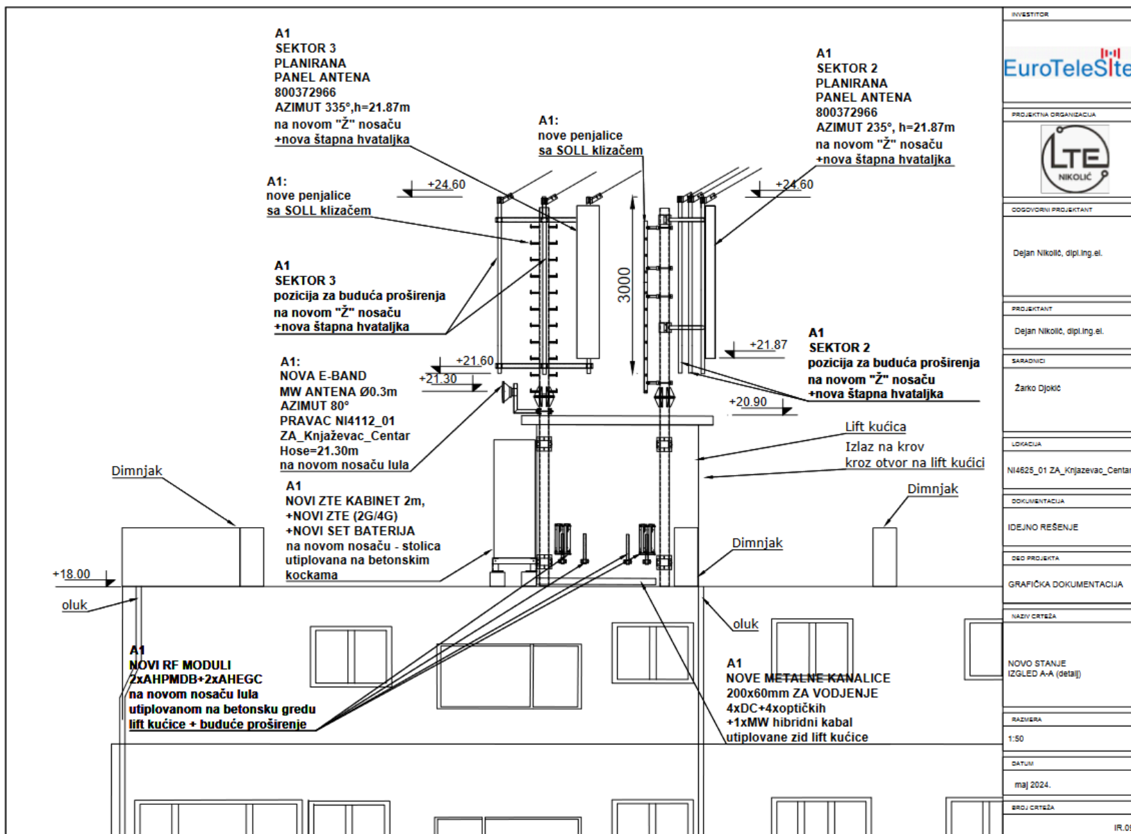
Слика 8.2. Идејно решење – изглед А-А (деталј) - ново стање
