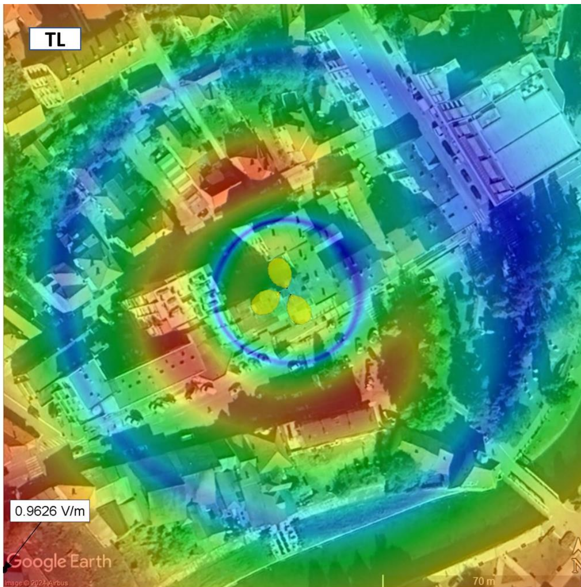
Слика 4.2. Јачина електричног поља на тлу када радио-систем GSM900 оператора А1 Србија ради максималним капацитетом
