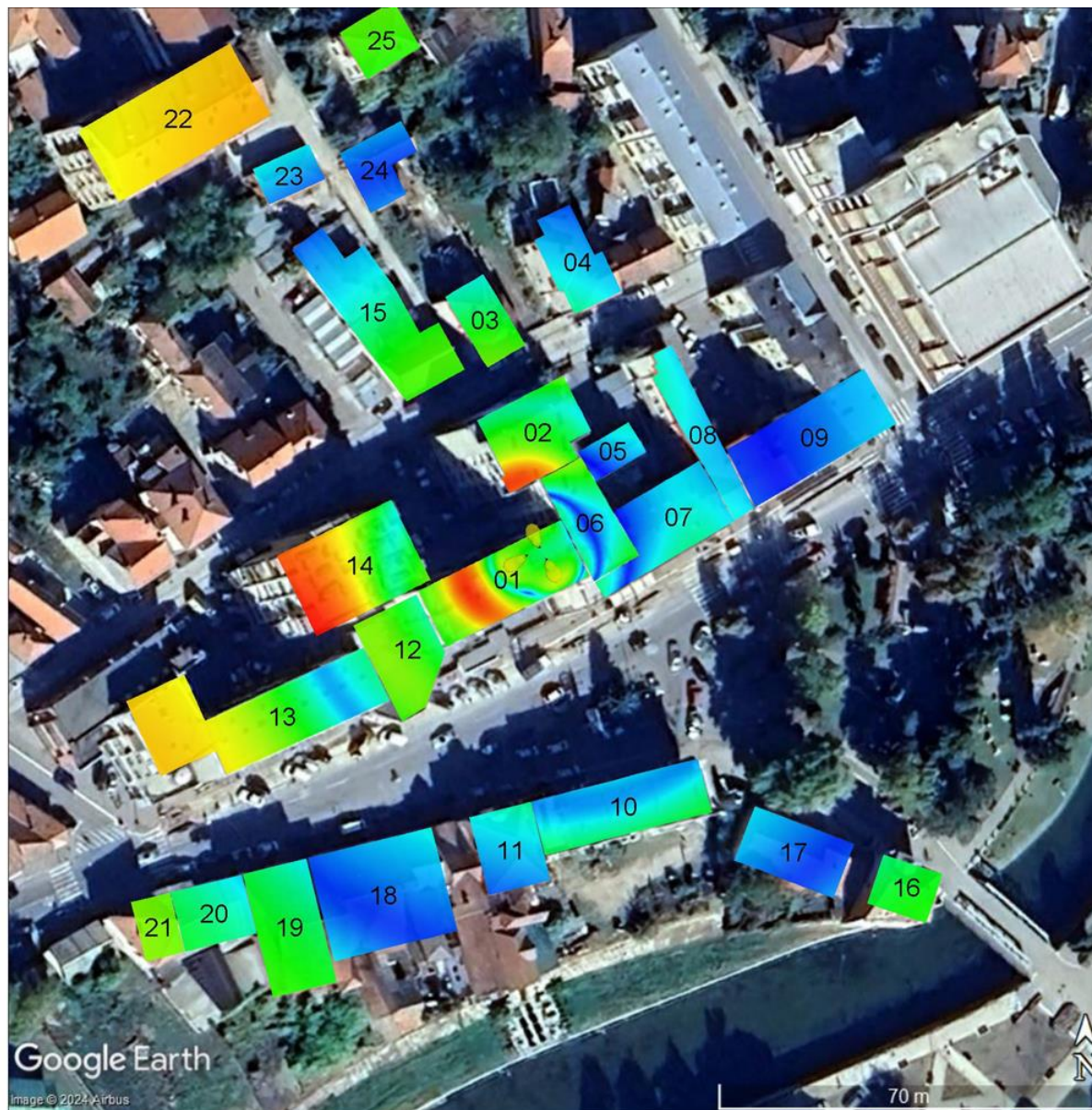
Слика 4.8. Јачина електричног поља унутар објекта када радио-систем LTE800 оператора А1 Србија ради максималним капацитетом
