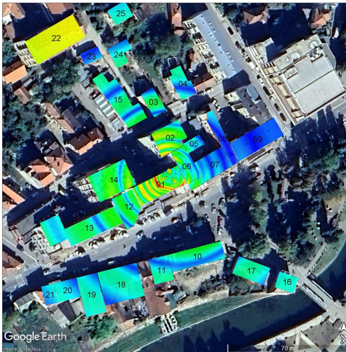
Слика 4.9. Јачина електричног поља унутар објеката када радио-систем LTE1800 оператора А1 Србија ради максималним капацитетом
