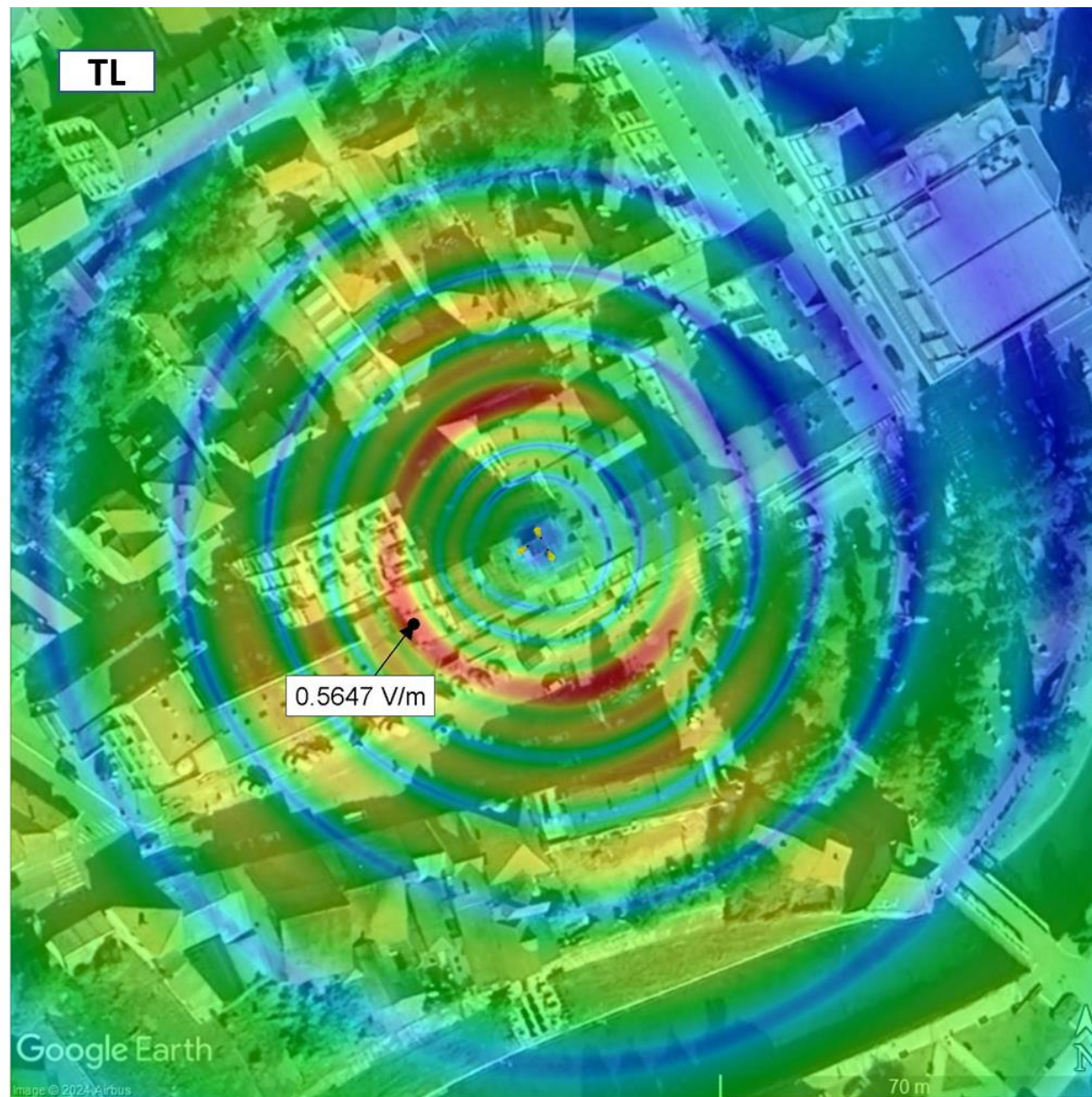
Слика 4.5. Јачина електричног поља на тлу када радио-систем LTE2100 оператора А1 Србија ради максималним капацитетом
