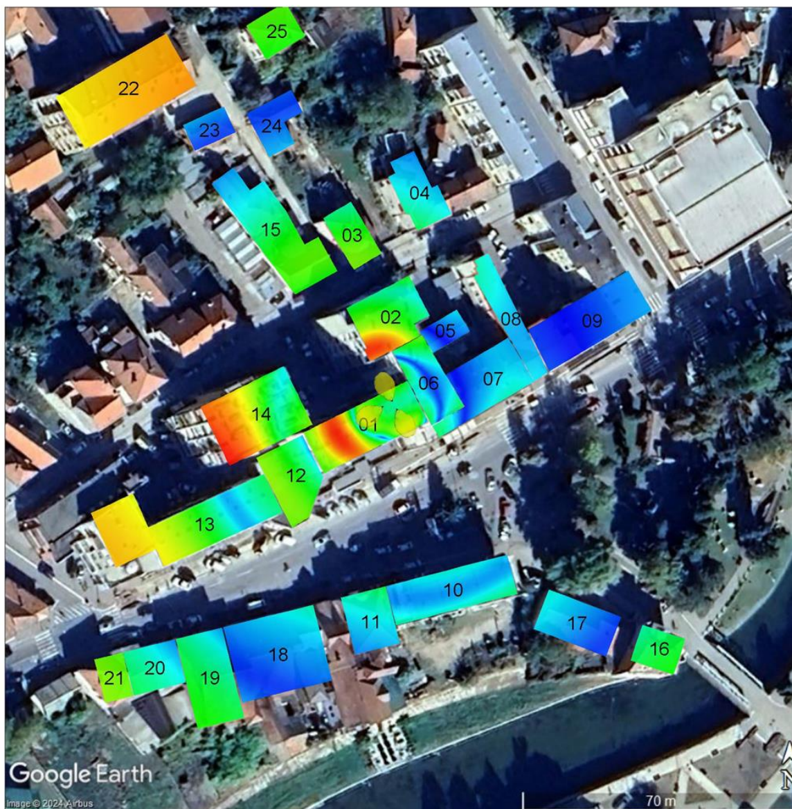
Слика 4.7. Јачина електричног поља унутар објеката када радио-систем GSM900 оператора А1 Србија ради максималним капацитетом
