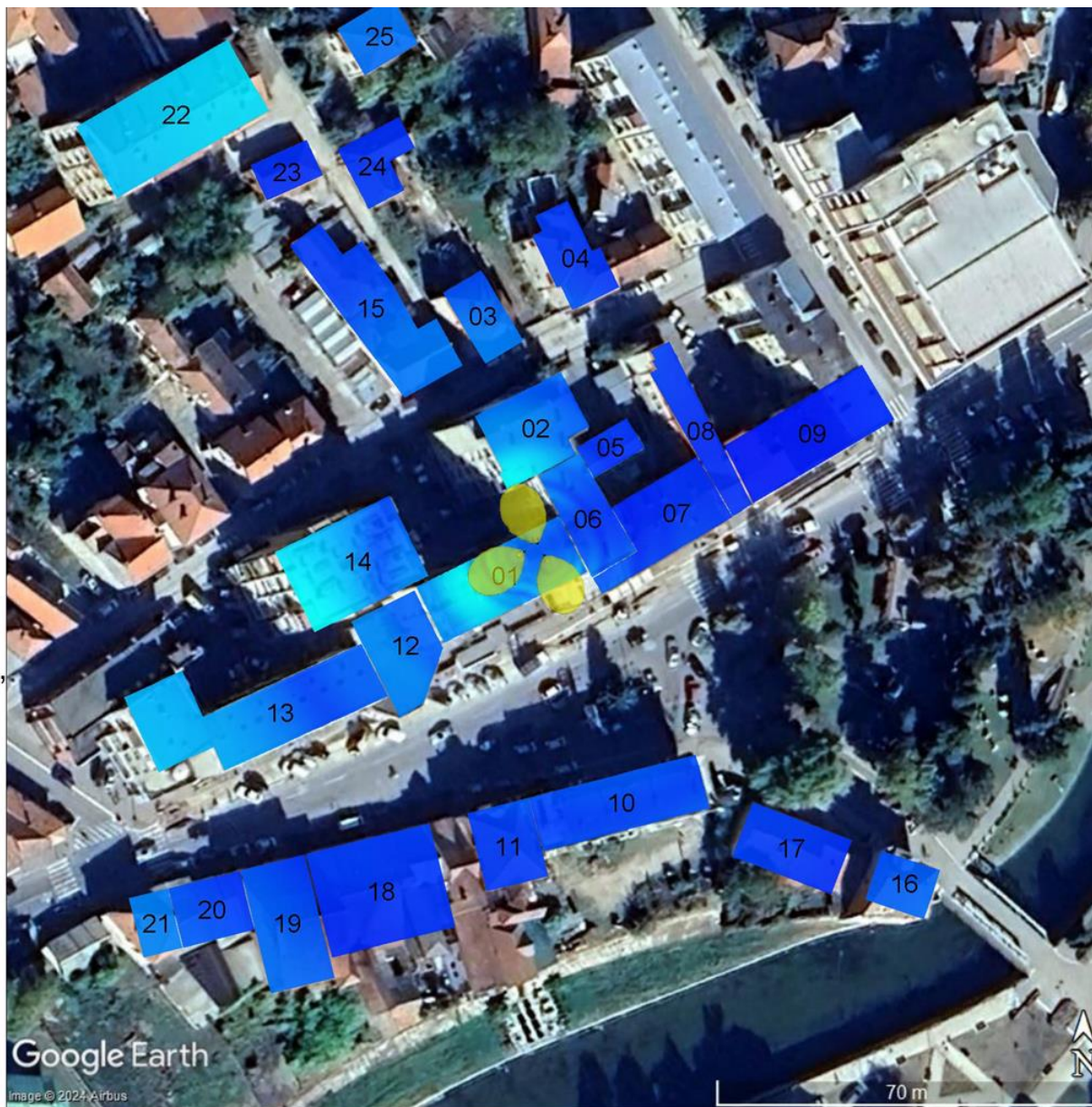
Слика 4.11. Фактор изложености унутар објекта када сви радио-системи оператора А1 Србија раде максималним капацитетом
