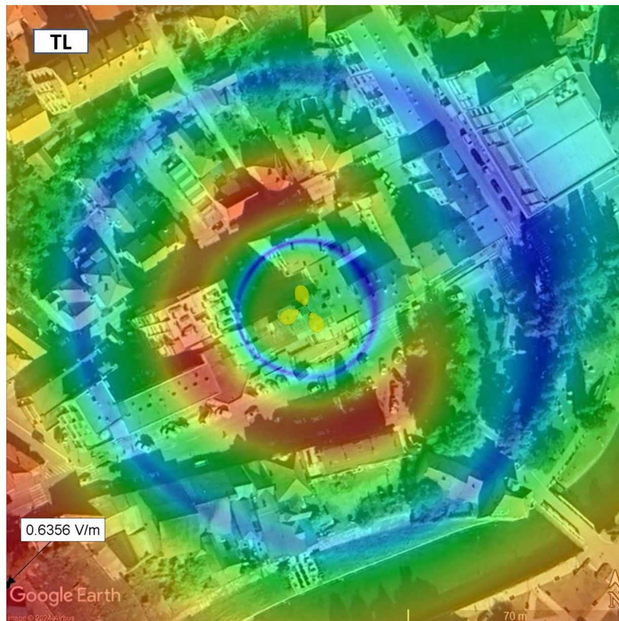
Слика 4.3. Јачина електричног поља на тлу када радио-систем LTE800 оператора A1 Србија ради максималним капацитетом
